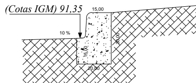
DETALLE CORDÓN SIMPLE H°
