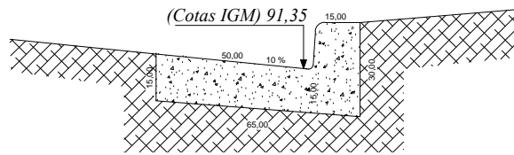
DETALLE CORDÓN CUNETA H°
