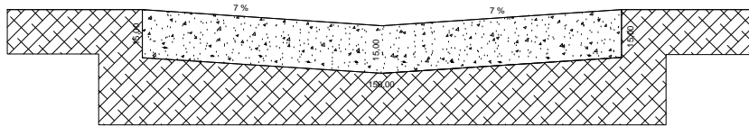
DETALLE BADÉN H°
